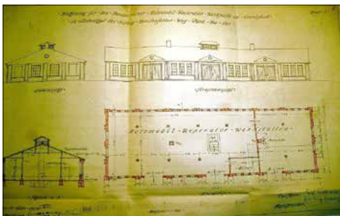
Plan 1924 Automobil-Reparatur-Werkstatt
